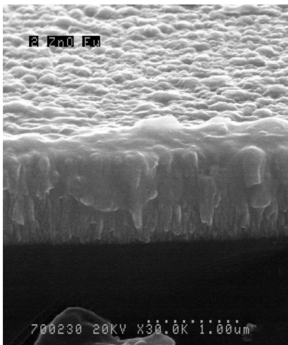
Сурет 4- Магнетронды тозаңдану әдісімен алынған ZnO:Eu үлбіршектерінің СЭМ бейнесі [6]
