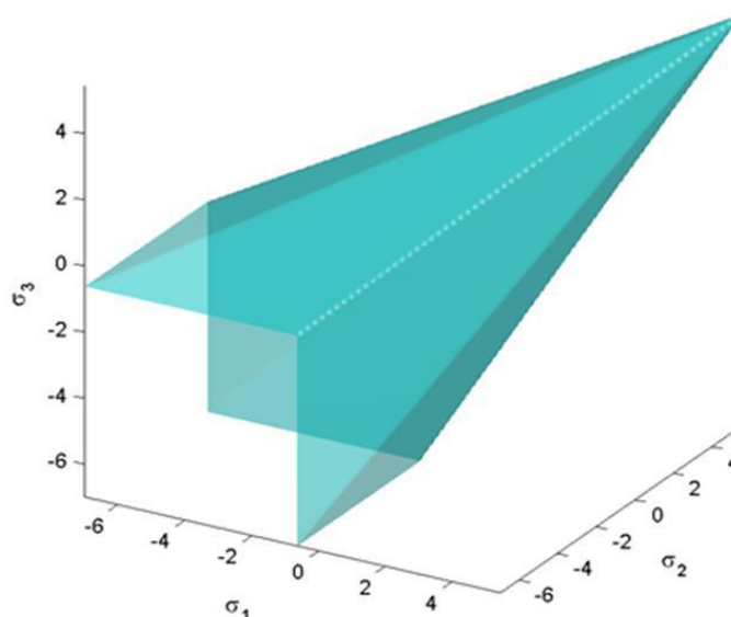
Рисунок 3- 3D модель поверхности
