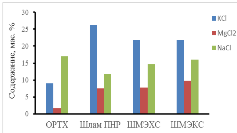
Рисунок 1 - Содержание KCl, MgCl 2 , NaCl в хлоридных отходах АО «УКТМК»
