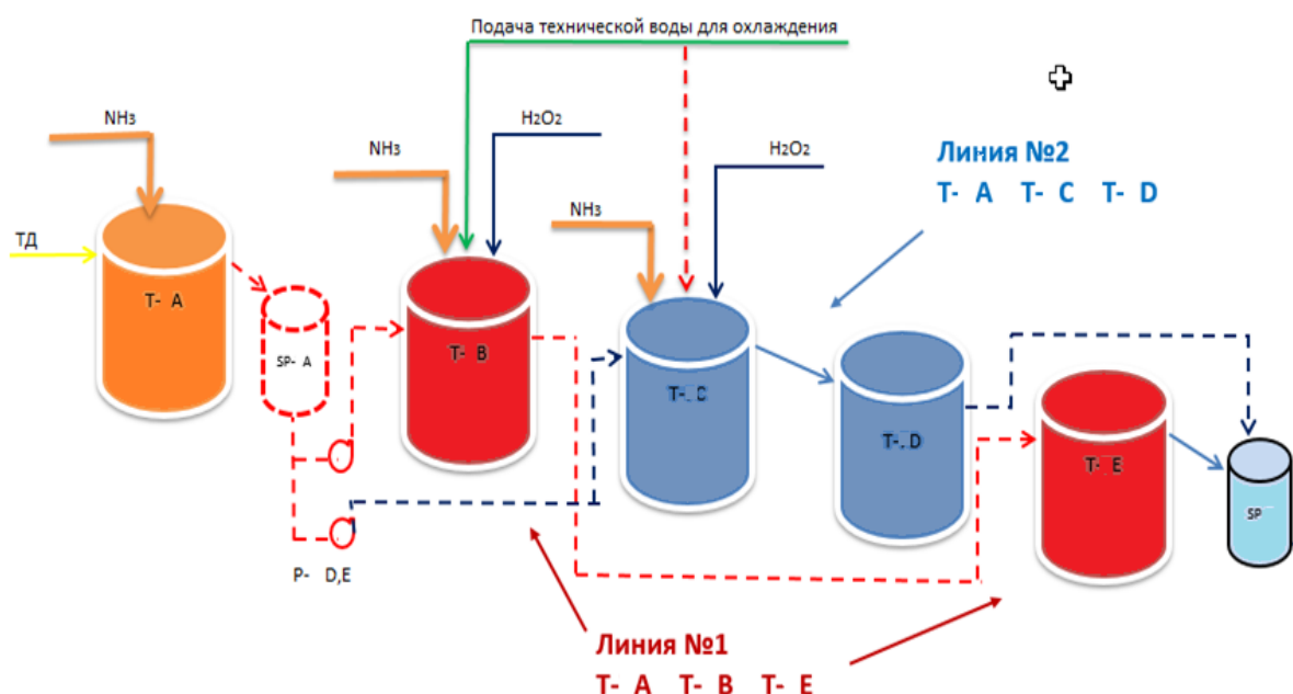
Рисунок 1. Схема каскада пероксидного осаждения
