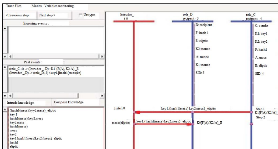
Рисунок 1. Результат проверки протокола средствами AVISPA: действия злоумышленника (Intruder) видны на графике внизу слева
