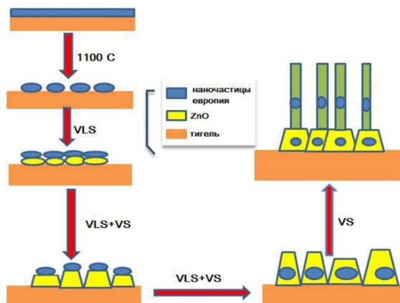
Сурет 2- Үшсатылы механизммен ZnO:Eu наноталшықтарының қалыптасуының схематикалық бейнесі [4]
