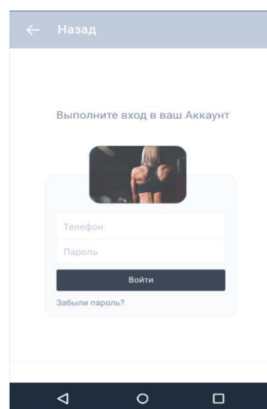
Рисунок 3. Окно авторизации
