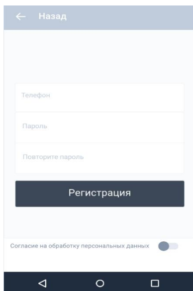
Рисунок 2. Окно регистрации
