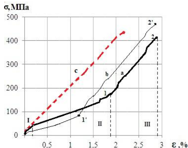
Рисунок 5 – Напряженно-деформированное состояние углепластика при скорости деформации 1 мм/мин: (а – образец №14; б – образец №26), при скорости деформации 20 мм/мин: (с – образец №14)
