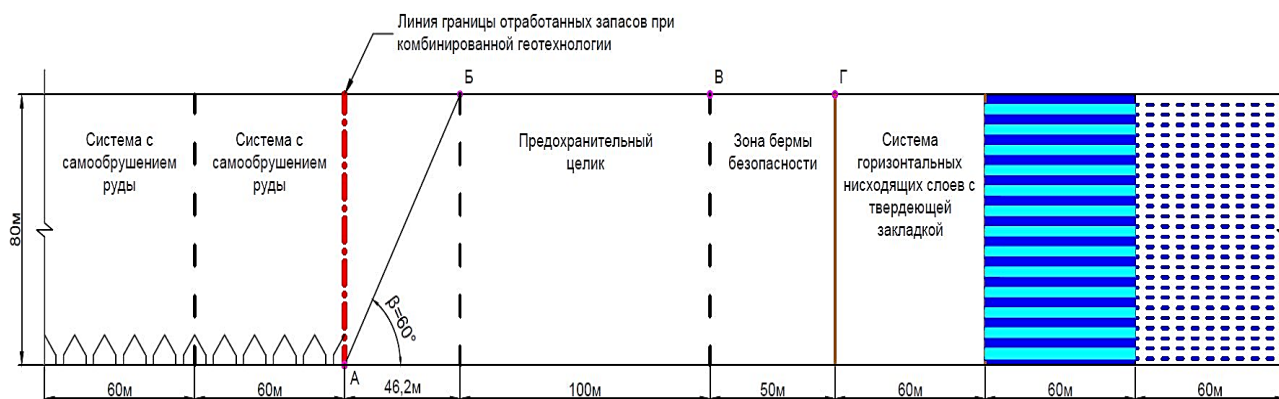
Рисунок 4 Схема бермы безопасности и предохранительного целика от влияния очистных работ при подземной добыче хромитов с применением комбинированной геотехнологии на глубоком горизонте шахт «ДНК» ДонГОКа
